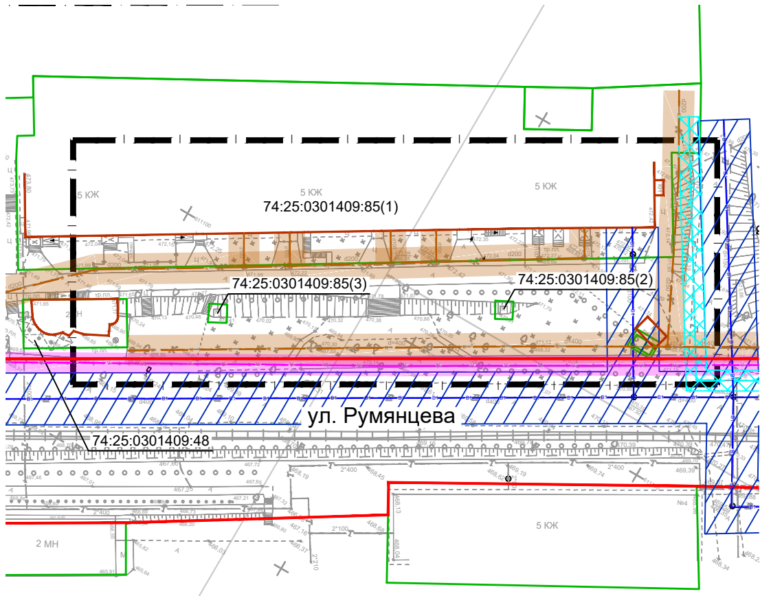
Лист 2. Чертеж материалов по обоснованию проекта межевания территории
